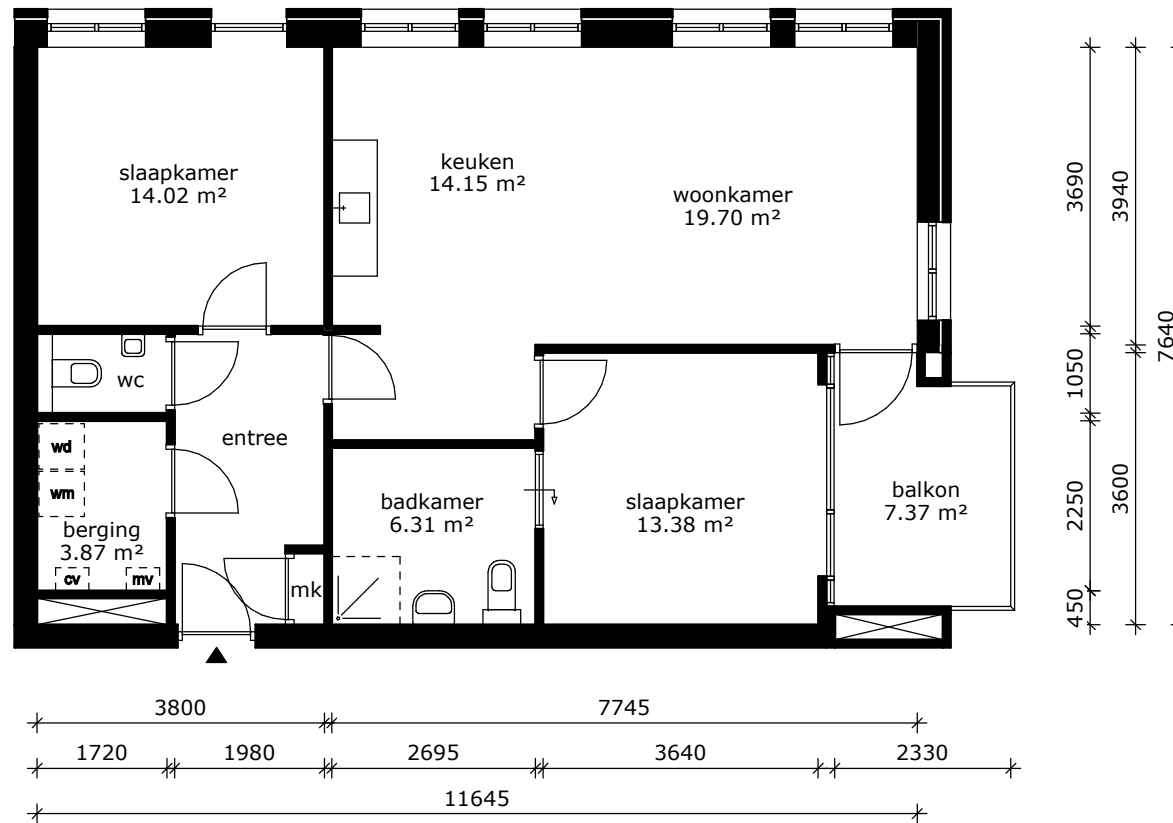
1e verdieping
